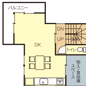
2階平面図
