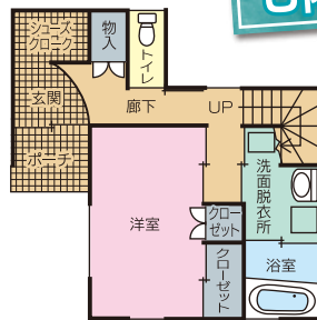
1階平面図
